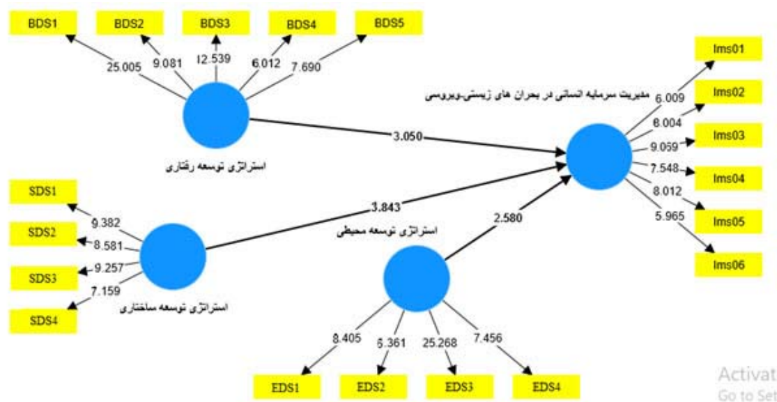
شکل ۲. ضرایب معناداری مدل ساختاری فرضیه‌های پژوهش
